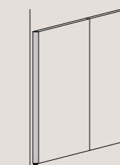
Sezione pannello standard / Section of standard panel
