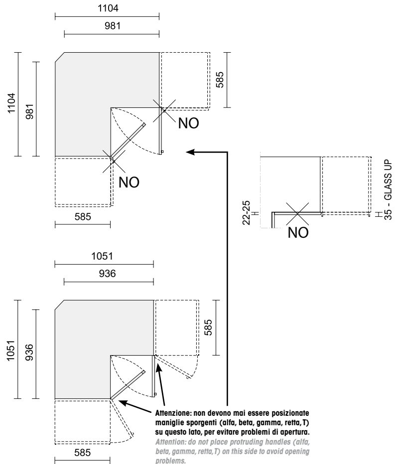
Pianta - Plan
